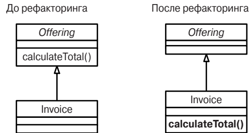
Рис. 2.1. Перенос метода из класса в подкласс
