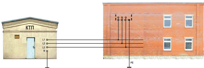
Система заземления ТТ (2)
